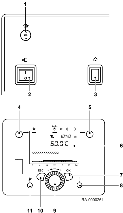
Рис. 3 Елементи управління
